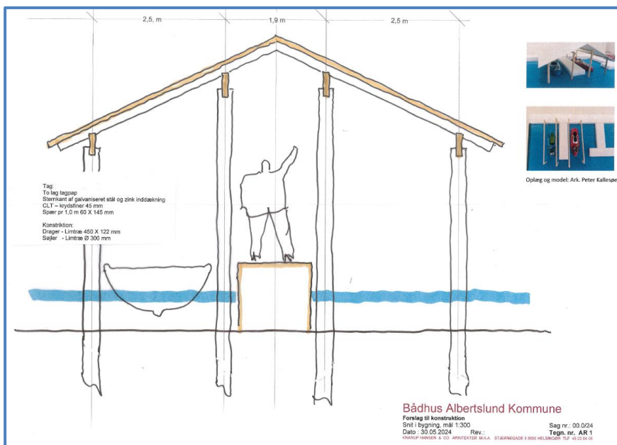
Visualisering af overdækningen ved Vallensbæk sø. Stolperne sættes ca. 1 meter i bunden.
